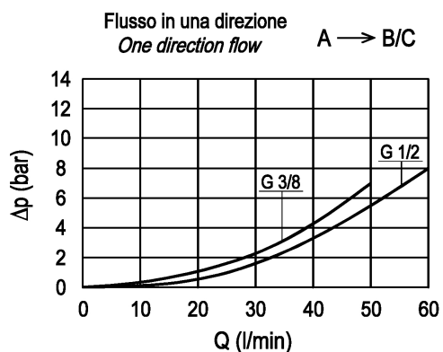
DIAGRAMMA PERDITE DI CARICO PRESSURE DROP CURVES
