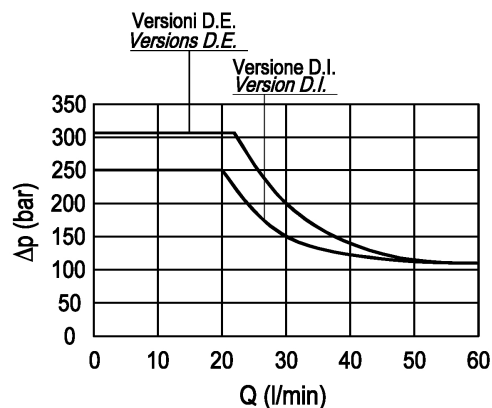
LIMITI DI FUNZIONAMENTO PERFORMANCE LIMITS
